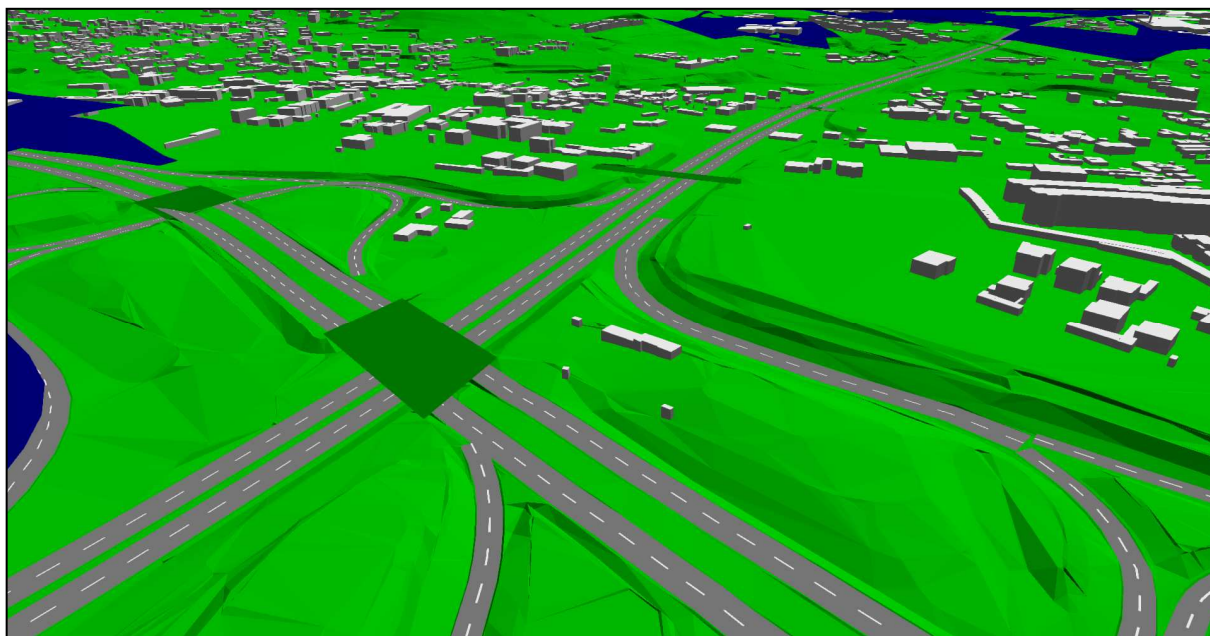
Figura 3.3 – Vista 3D da zona do nó da A1 com a A41
