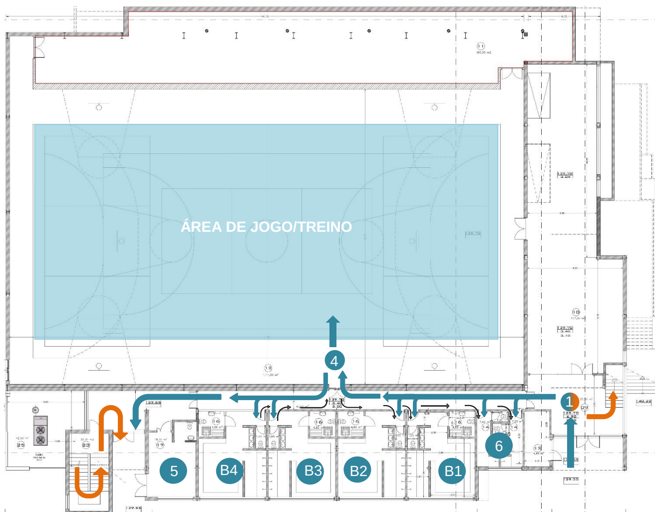
Imagem 1 – Fluxos de circulação (piso 0).
